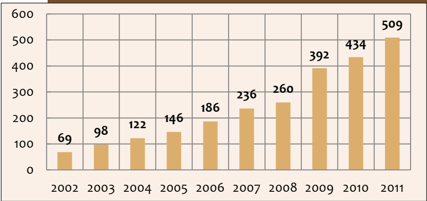
Գազի բաշխիչ գործող ցանցի միագիծ երկարությունը Արագածոտնի մարզի գյուղական վայրերում (կմ)
